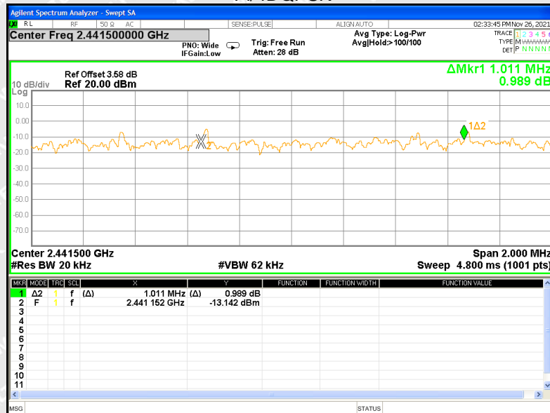
Pi/4DQPSK
