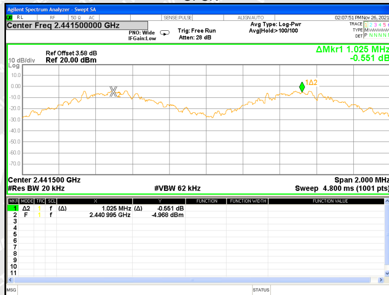
Pi/4DQPSK
